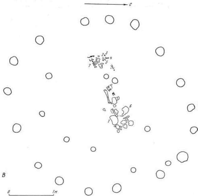
В — план погребения; 1 — обработанный плоский камень; 2 — каменный терочник; 3 — бронзовый наконечник; 4 — обуглившийся деревянный гробчик; 5 — фрагмент наделки из бронзы; 6 — обуглившаяся ткань; 7 — обуглившееся дерево
